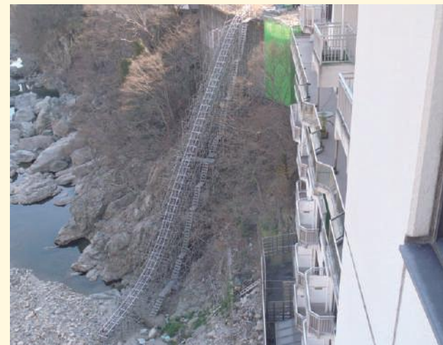
道路脇から護岸ヘレールを設置
